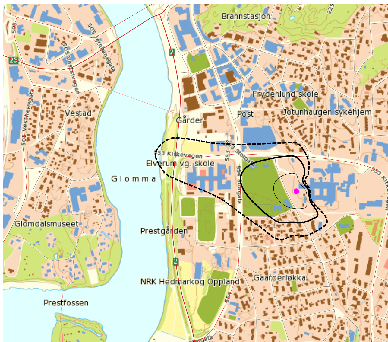
Figur 9-1. Kartleggings- og tiltaksgrenser i henhold til forurensingsforskriften. Kotene viser L_{Aeq24h} 51, 54 og 61 dBA. M 1:10 000.
