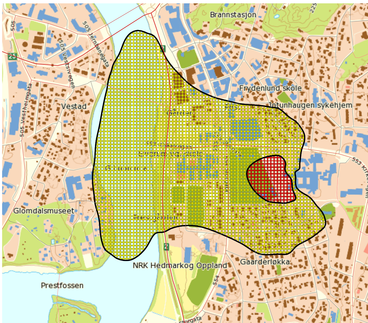
Figur 8-3. Støysonekart etter T-1442/2012 for landingsplassen. M 1:10 000.
